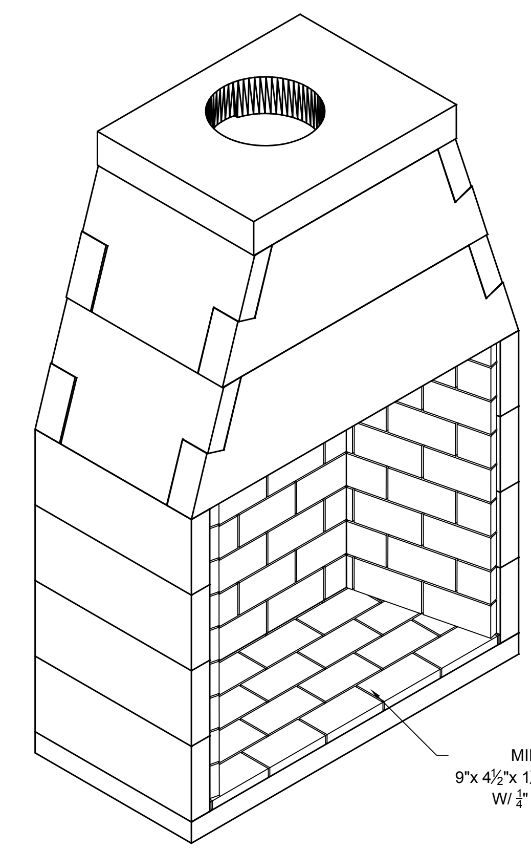
ISOMETRIC VIEW SCALE: N.T.S.
